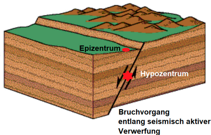
Abbildung 5: Skizze (nicht maßstabsgerecht) zur Beschreibung der Entstehung und Auswirkungen eines Erdbebens (der rote Stern markiert das Hypozentrum) aufgrund der Bewegung an einer aktiven geologischen Störung / Verwerfung (durch Pfeile markiert).
